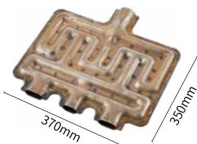
冲压铁火管
