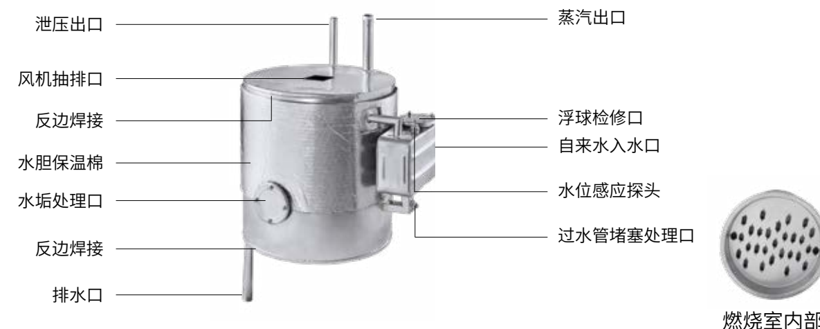
A1 蒸汽机内胆各型号（包含水垢处理口、保温棉、拉伸成型承压副水箱）
