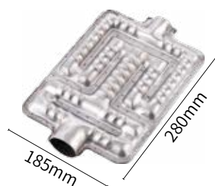
冲压火管
