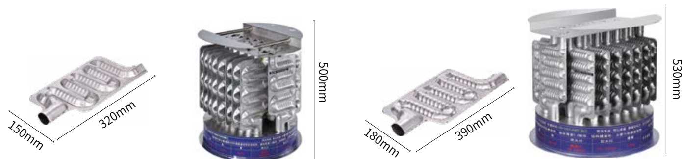
菱形 6 层火管
