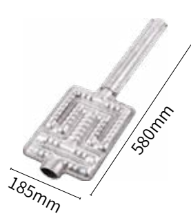
冲压火管
